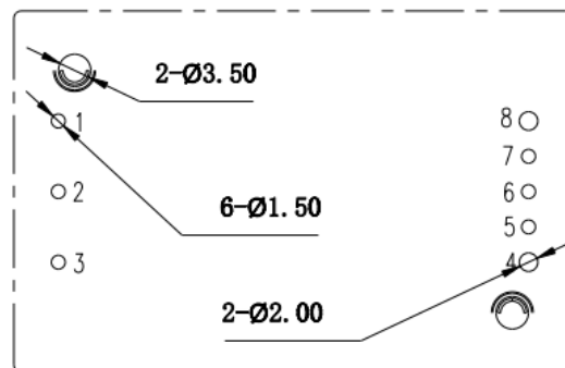
推荐PCB开槽尺寸
