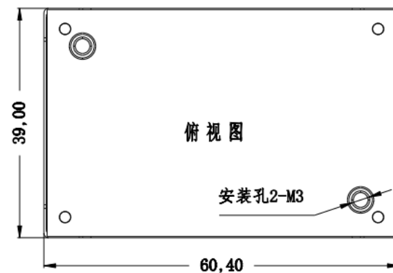
标准型 60.4*39*12.7mm
